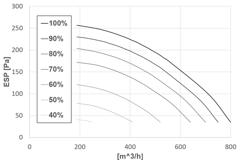
Figura 7 - Pressione statica esterna vs portata d'aria a varie velocità del ventilatore.
