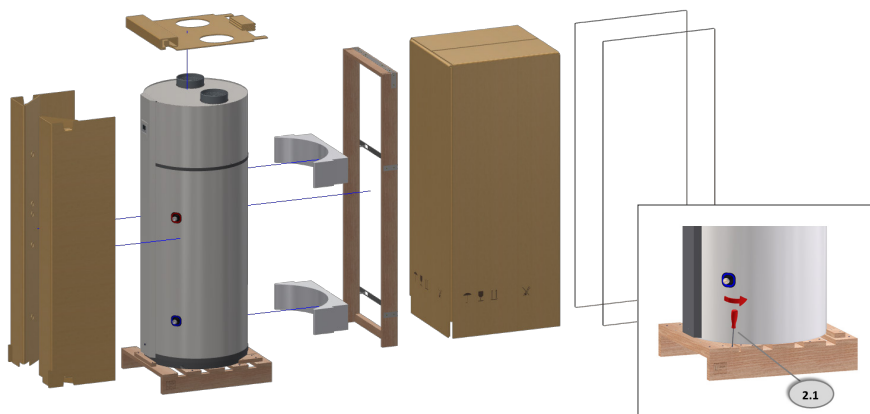
Figura 10 - Sequenza di montaggio
