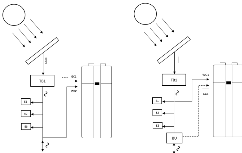
Figura 20 - Installazione PV 1: segnale di controllo da inverter. Installazione PV 2: Segnale di controllo da misuratore di energia.
