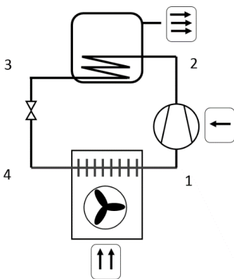
Figura 1 - Principio della pompa di calore
