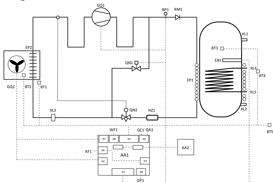
Figura 3 – Diagramma di Processo e Strumentazione
