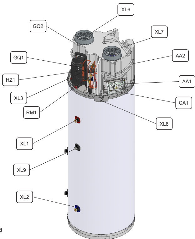
Figura 4 - Configurazione del circuito frigorifero e dei componenti principali
