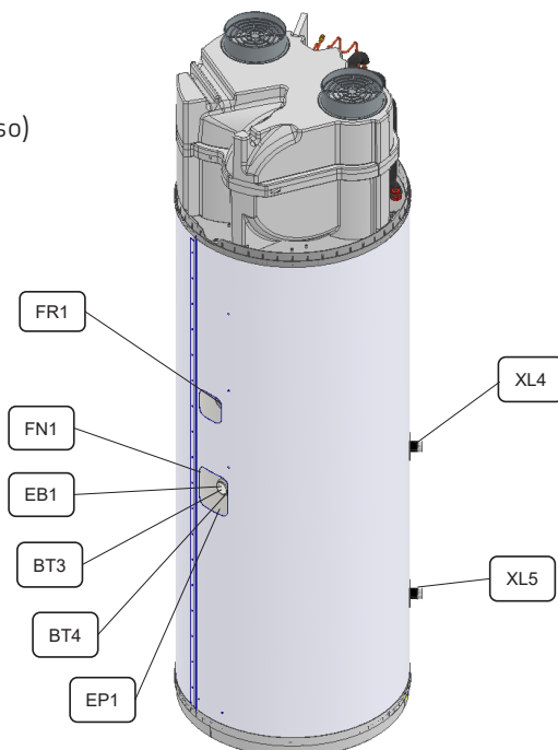
Figura 5 - Configurazione del serbatoio, condensatore e relativi componenti
