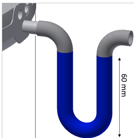
Figura 12 - Scolo condensa
