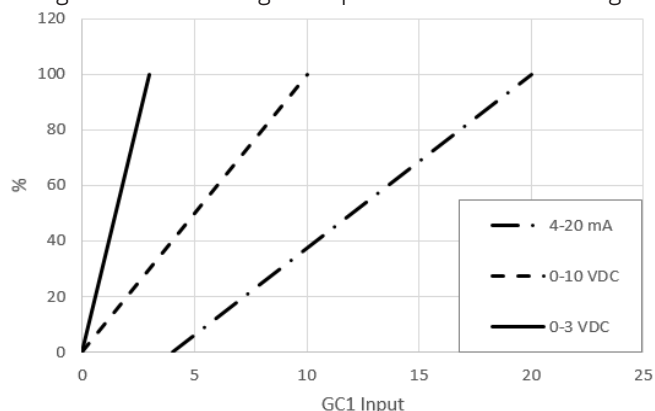
Figura 21 - Tabella di conversione del segnale d'ingresso del controllore a percentuale
