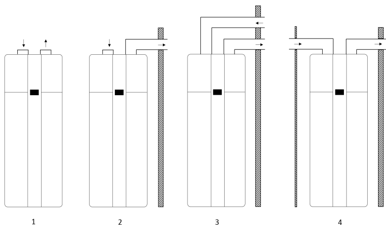
Figura 13 - Configurazione dei condotti dell'aria
