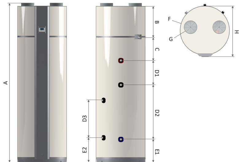
Figura 6 - Dimensioni
