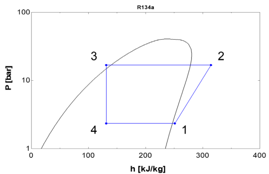
Figura 2 - Diagramma Pressione-Entalpia
