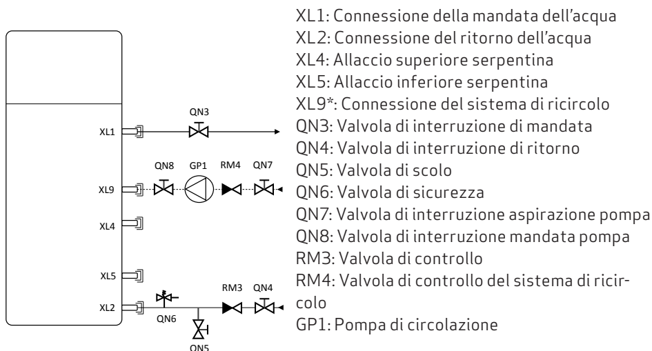
Figura 11 - Diagramma delle connessioni idrauliche raccomandate
