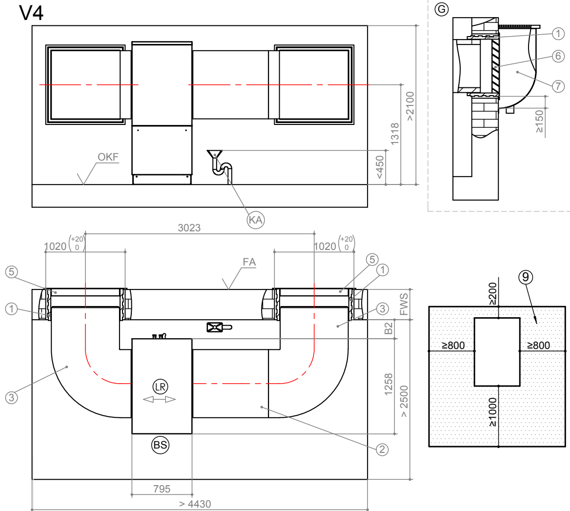
Aufstellungsplan V4
