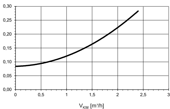
Δpmax [bar]
