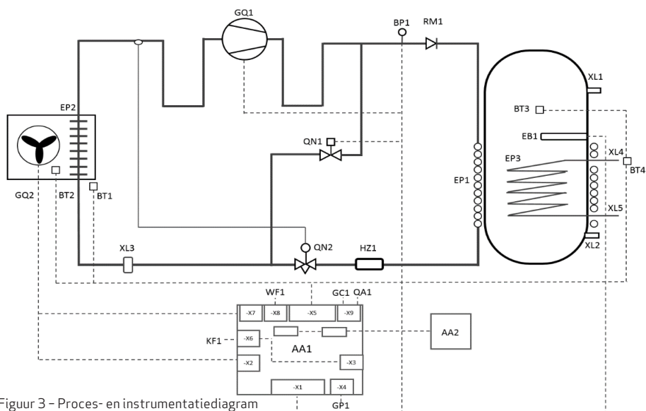
Figuur 3 – Proces- en instrumentatiediagram
