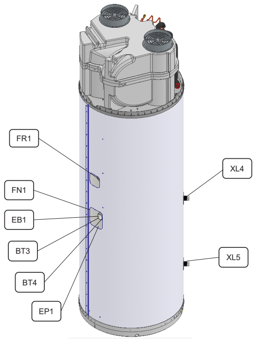
Figuur 5 - Het ontwerp van het reservoir, de condensator en bijbehorende onderdelen
