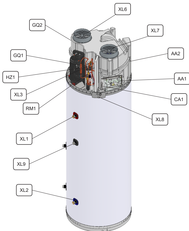
Figuur 4 – Ontwerp koelcircuit en de hoofdcomponenten
