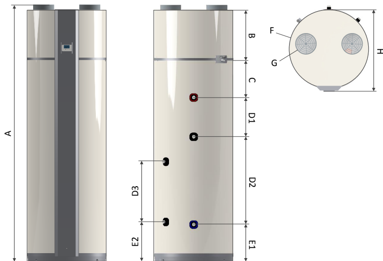
Figuur 6 - Afmetingsgegevens
