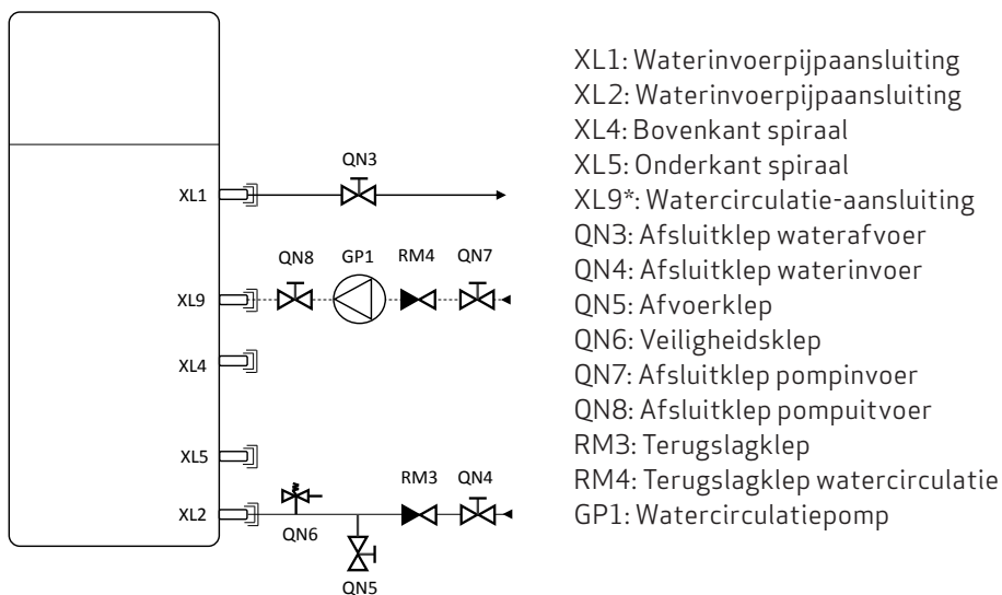
Figuur 11 – Schema van voorgestelde watercircuitaansluitingen
